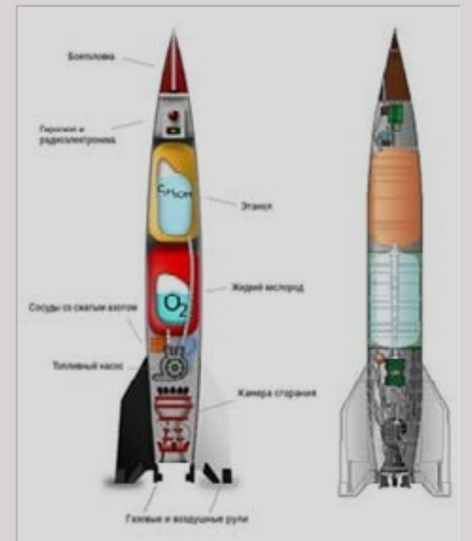
Ракеты V-2 (Vergeltungswaffe-2) (слева) и P-1 (справа)
